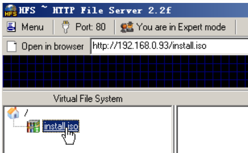
图 3.24. hfs_2
