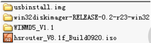
图 3.59. 准备文件
